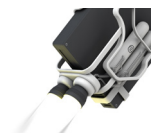
O&O Defrag
